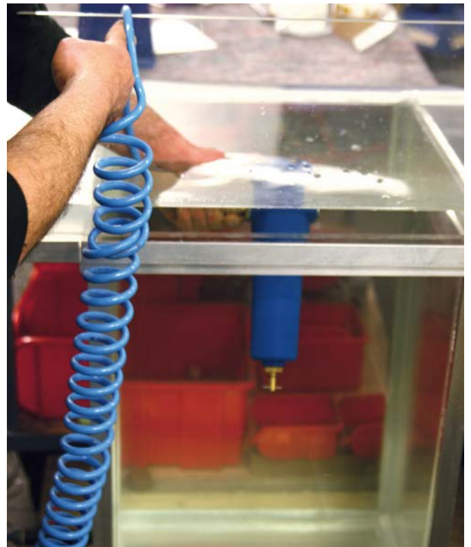
Dichtigkeitsprüfung jedes Druckluftfilters
