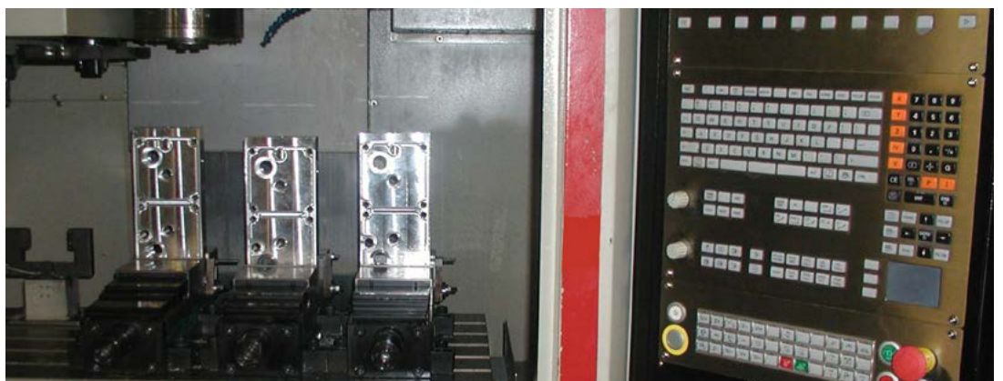
CNC-Fräsen von Aluminiumbauteilen für die Adsorptionstrockner-Baureihe AT-APN.
