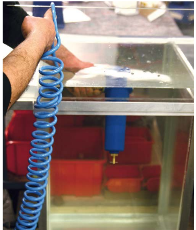
Ensayos de fugas para filtros de aire comprimido
