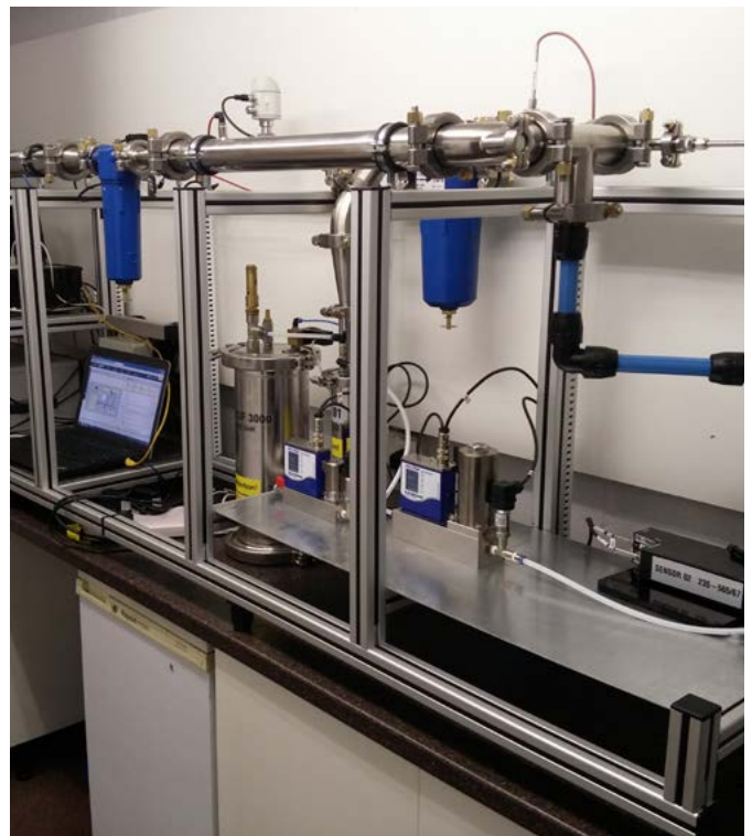
Estación de prueba de elementos filtrantes, incluyendo contador de partículas
